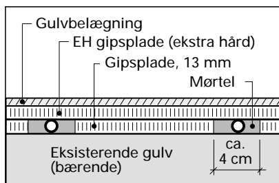
Gipspladegulv anvendt ved renovering.
