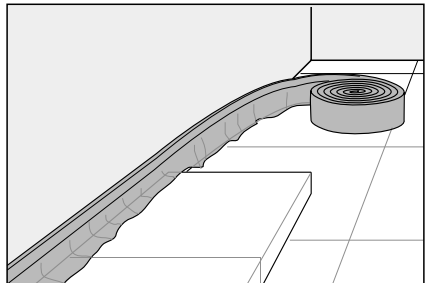
Montering af kantisolering.
