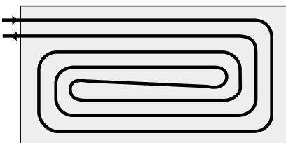
In-line-streng med dobbelt rørføring
