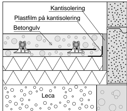
Placering af kantisolering til et rågulv.
