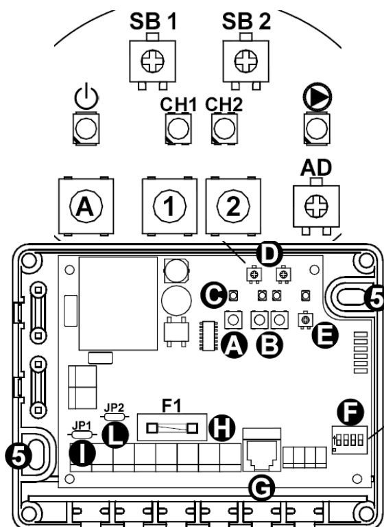
Fig. 2: Basisenhedens printkort med div. Klemmer, sikring, DIP-switch.
